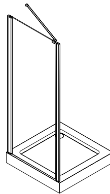
Seitenwand anschlagseitig 1 × C5W1A90 (Breite 900 mm)
