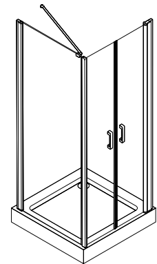
Eckdusche 2 × CP245 (Breite 900 mm) + 1 × C5W1A90 (Breite 900 mm)
