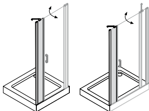
zur schließseitigen Kombination mit den Nischentüren CP1 und CP2A
