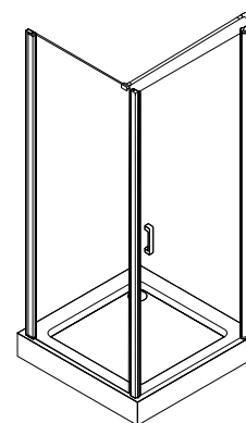
■ Eckdusche 1 × CE290 (Breite 900 mm) + 1 × CSW1590 (Breite 900 mm)
