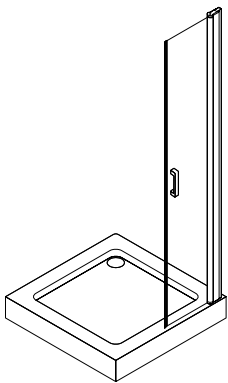
Pendelhälfte ohne Festelement 1 × CP245 (Breite 450 mm)
